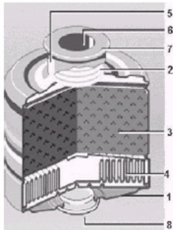
Bild 13: Kombinationsfilter
