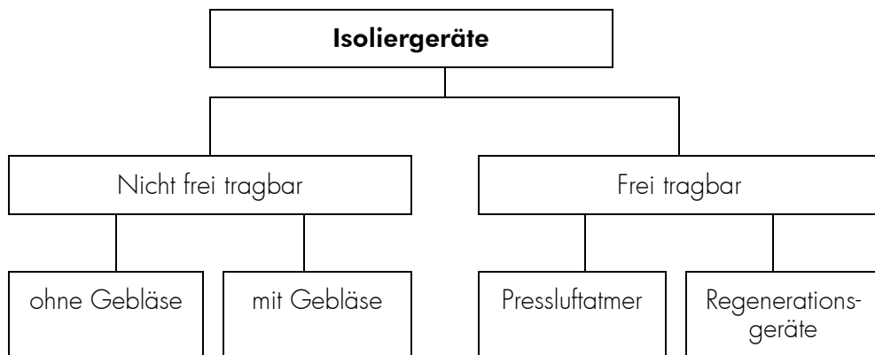
Bild 3: Unterteilung der unabhängig von der Umgebungsatmosphäre wirkenden Atemschutzgeräte
