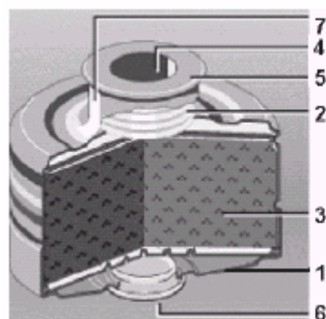
Bild 12: Gasfilter
