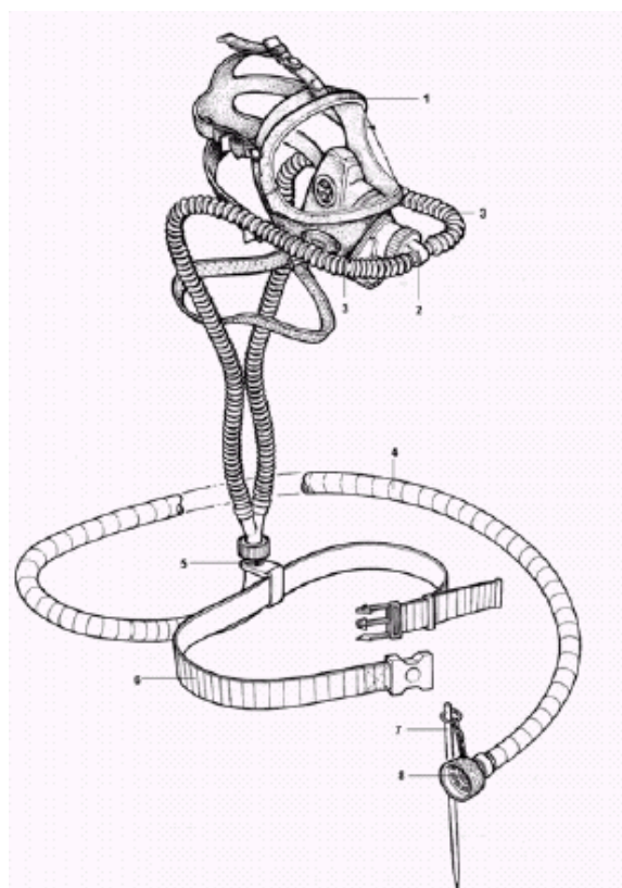
Bild 21: Frischluft-Saugschlauchgerät
