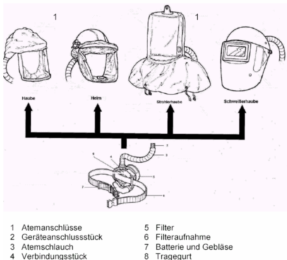
Bild 18: Filtergerät mit Gebläse und Haube oder Helm und einem Hauptfilter
