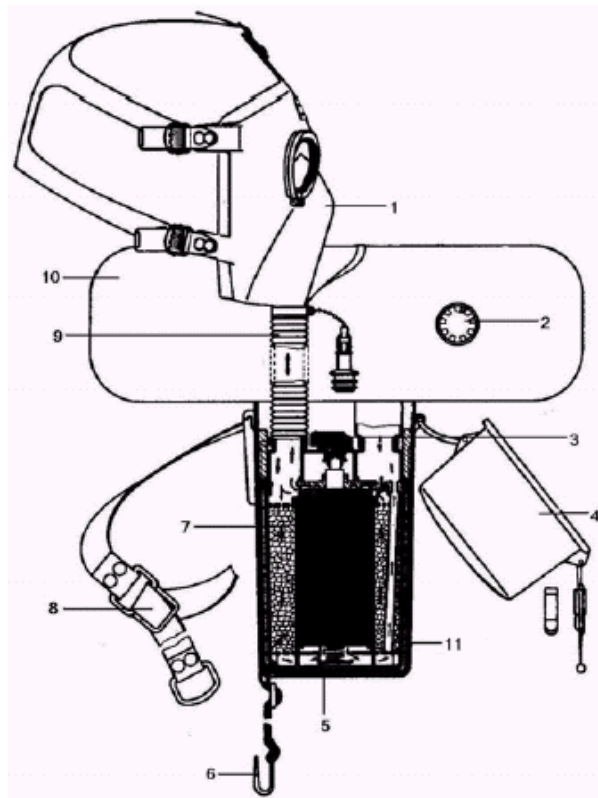
Bild 32: Chemical-Sauerstoff(NaClO 3 )selbstretter
