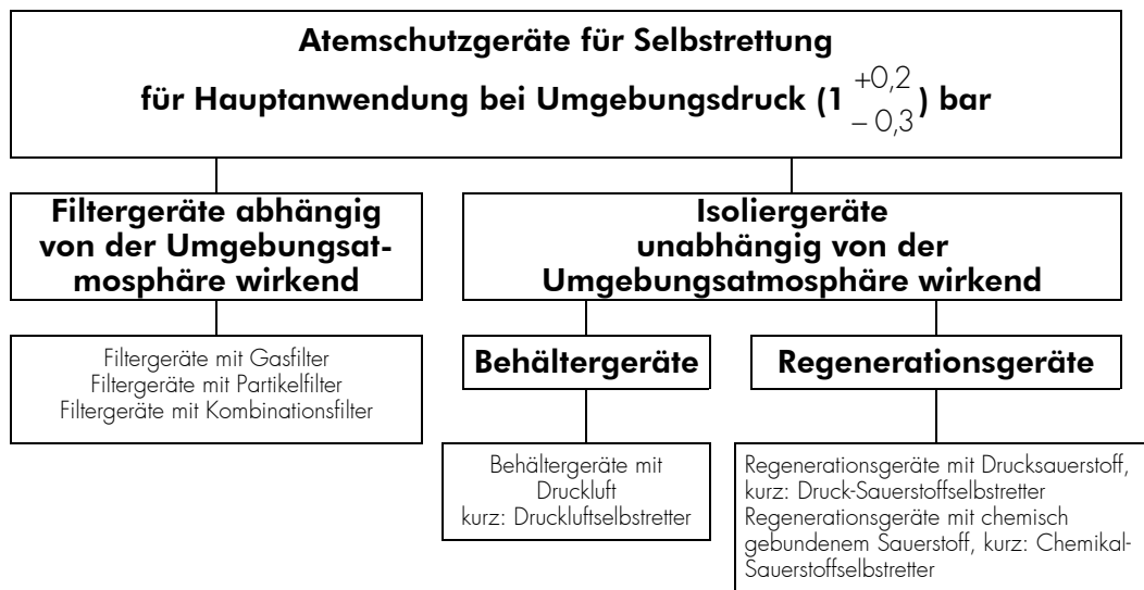
Bild 6: Einteilung der Atemschutzgeräte für Selbstrettung und Flucht
