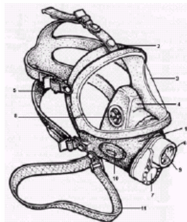
Bild 8: Vollmaske
