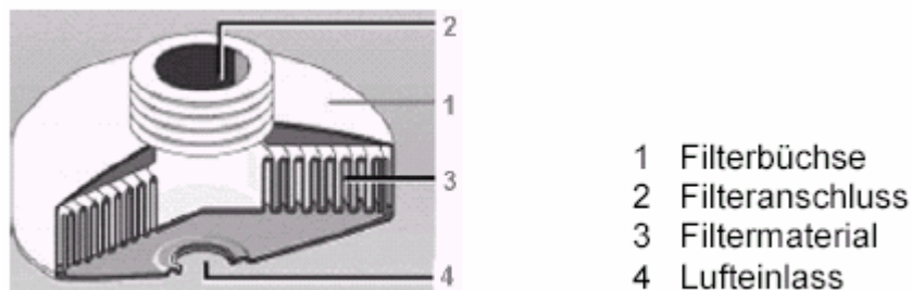
Bild 11: Partikelfilter
