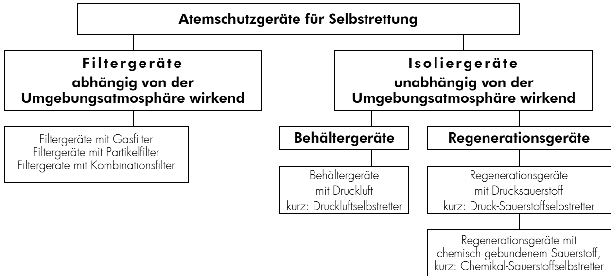
Bild 28: Einteilung der Atemschutzgeräte für Selbstrettung
