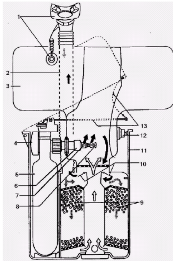
Bild 30: Druck-Sauerstoffselbstretter
