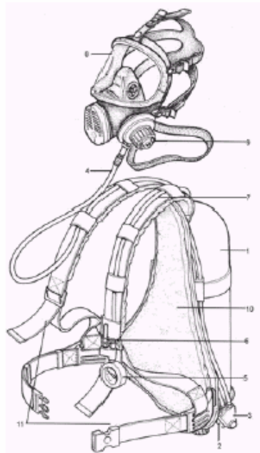
Bild 24: Behältergerät mit Druckluft
