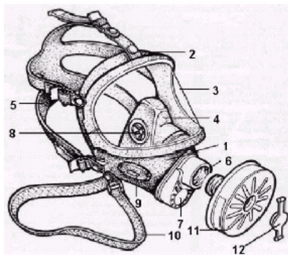
Bild 16: Vollmaske mit Partikelfilter
