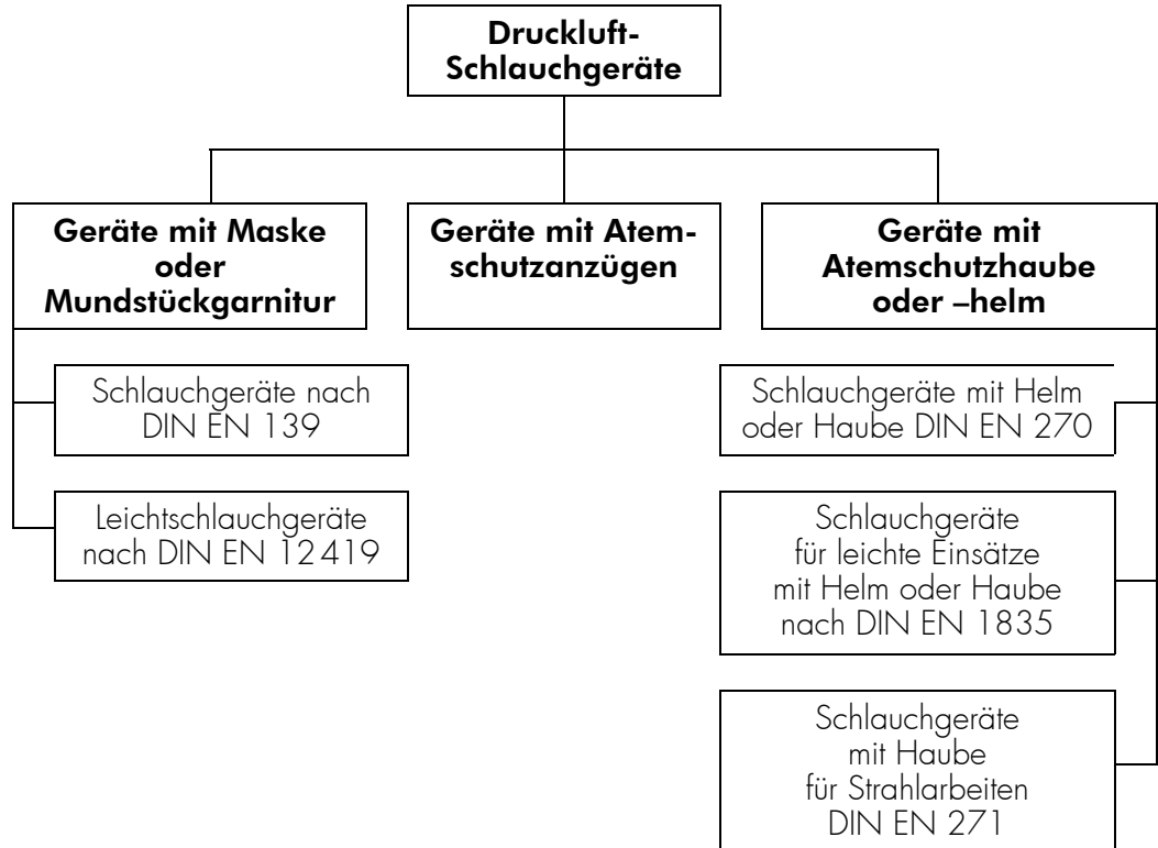
Bild 22: Einteilung der Schlauchgeräte
