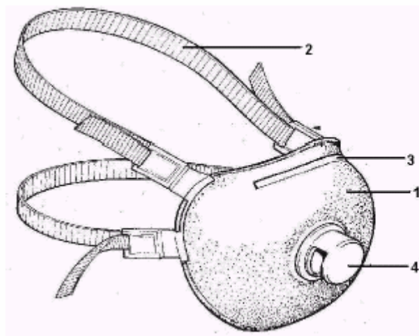
Bild 15: Partikelfiltrierende Halbmaske
