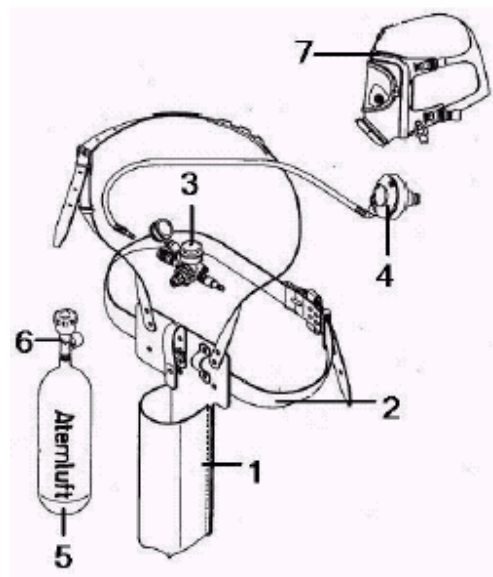
Bild 29: Druckluftselbstretter
