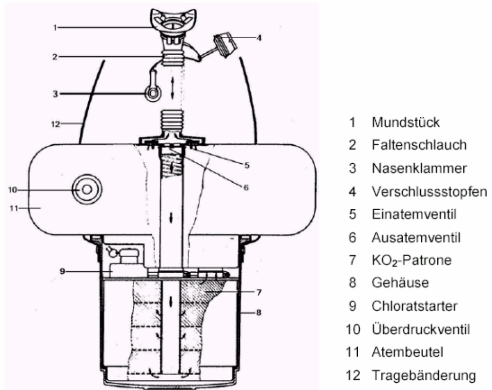
Bild 31: Chemikal-Sauerstoff(KO 2 )selbstretter
