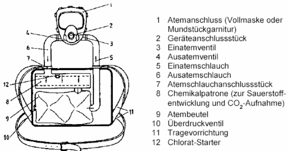
Bild 26: Regenerationsgerät mit Chemikalsauerstoff ( \text{KO}_2 )
