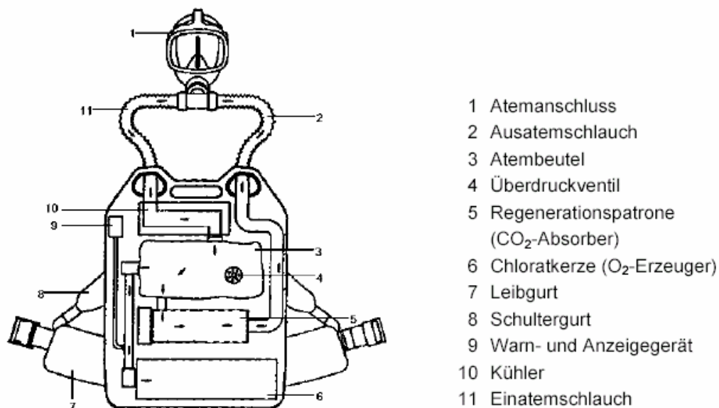
Bild 27: Regenerationsgerät mit Chemikalsauerstoff (NaClO 3 )
